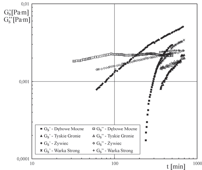
Rys. 2. Zależność G_s' i G_s'' badanych piw w funkcji czasu t .
